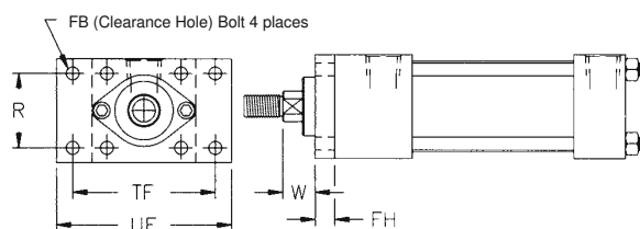
Mount Code F1 NFA MF1
